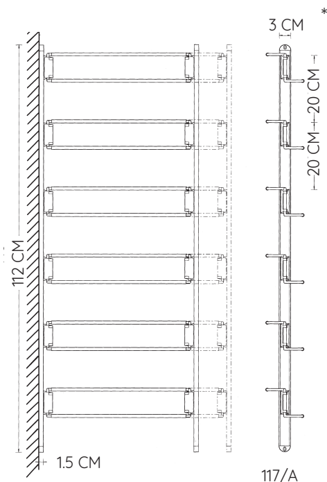
Laterale. *applicato sul guida / Side application on runner
